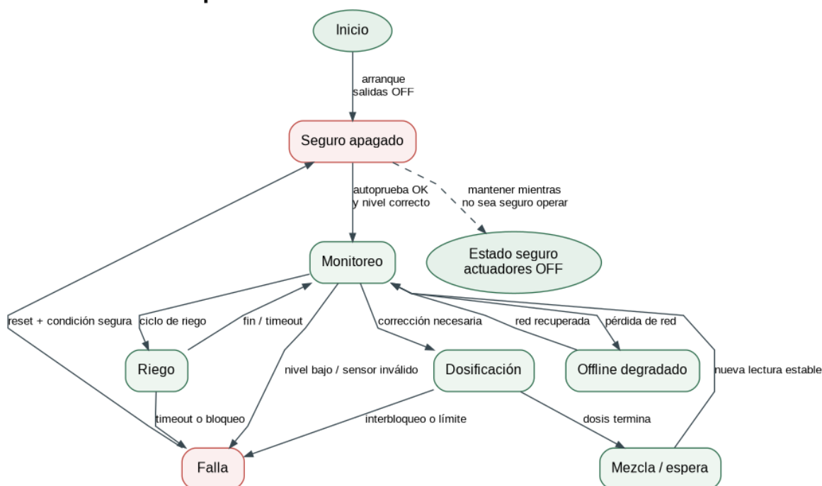
Figura 6. Máquina de estados propuesta para el ESP32.
