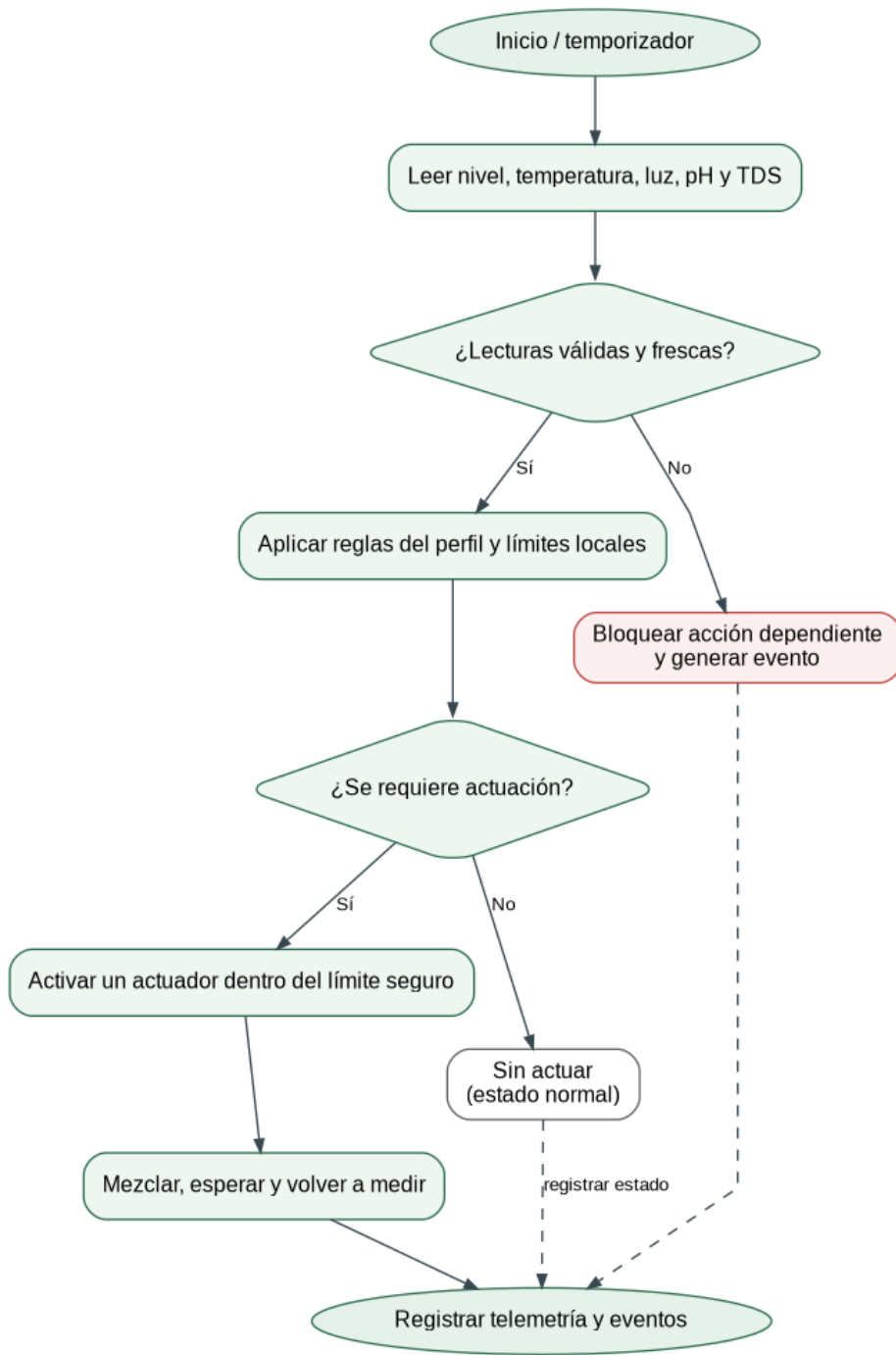
Figura 3. Actividad del ciclo local de adquisición y control.
