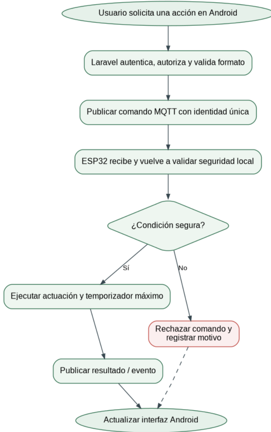
Figura 4. Actividad de una orden remota segura.
